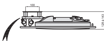
Détail de la fixation / Befestigungsdetail
